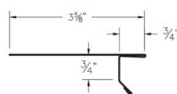
⑥⑩ Drip Edge (DEcc)
