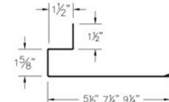
②② Door Trim (JTcc725 or JTcc925)
