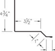
⑧ Universal Sidewall (SWcc)
